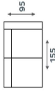
2-ZITS ARM RECHTS
